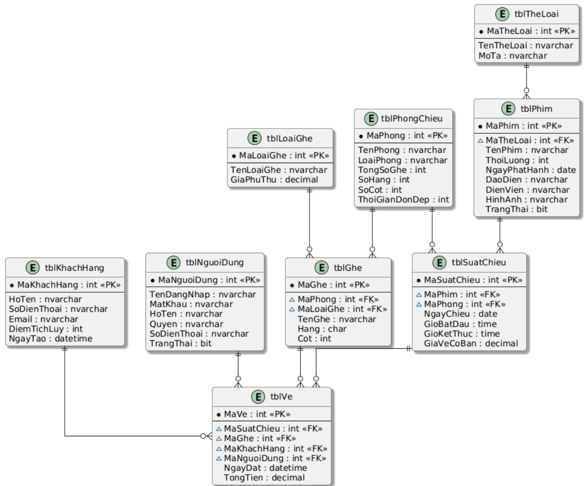
Hình 2.3. Mô hình liên kết
