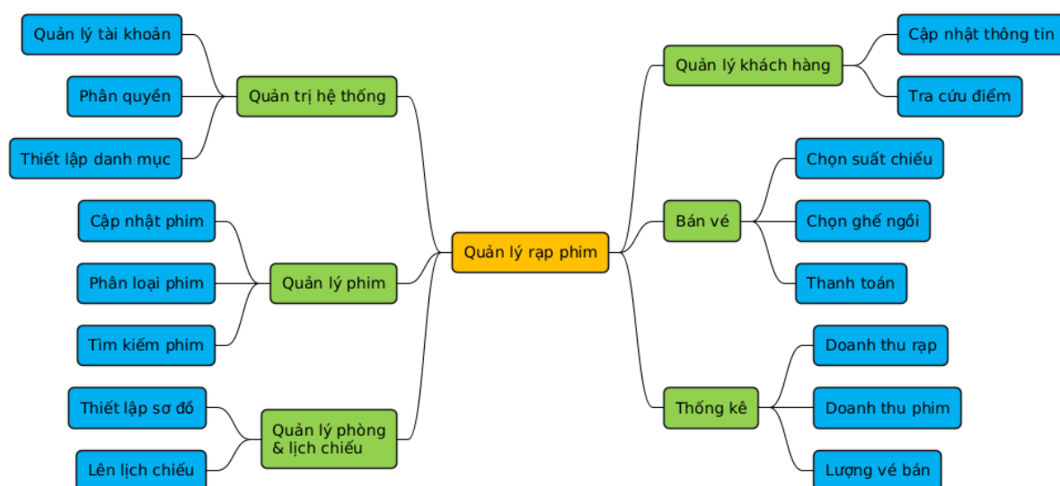
Hình 2.2. Sơ đồ phân cấp chức năng của hệ thống
