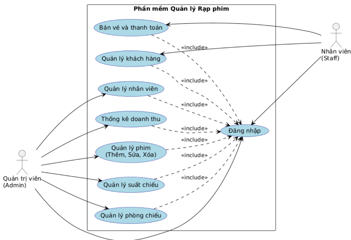
Hình 2.1. Sơ đồ UseCase tổng quát
